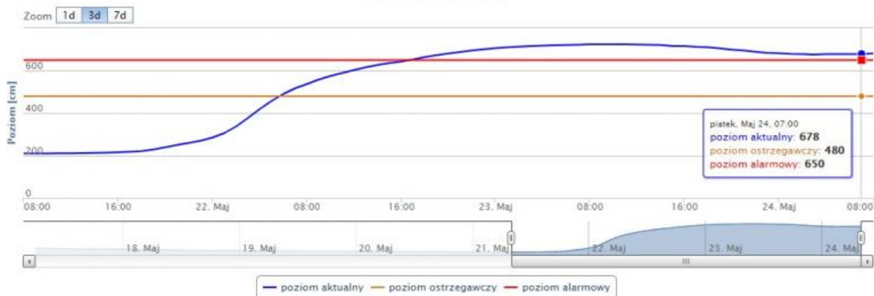
Wodowskaz: MIELEC 2
