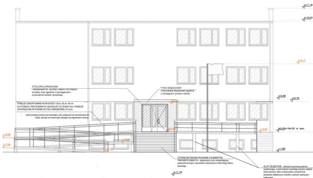
ELEWACJA WSCHODNIA
